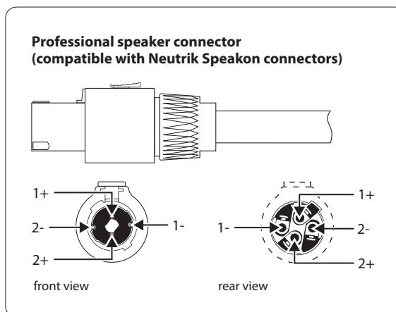
Рис. 1.3: Штекер Speakon
